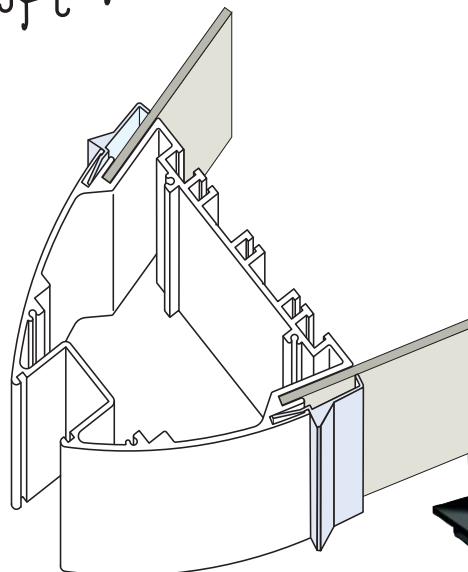
Détail du profilé 157
